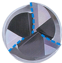
突込み加工時のSUS304切りくず形状
